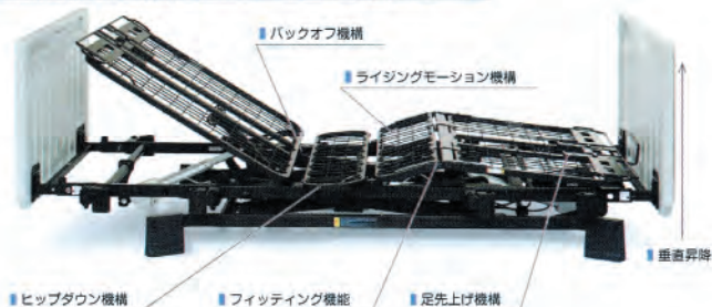
ヒップダウン機構
